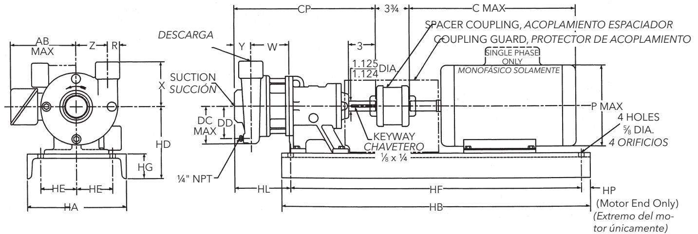
Pump Dimensions and Weights Peso y dimensiones de la bomba (la dimensión "HL" está determinada por la bomba y el motor)
